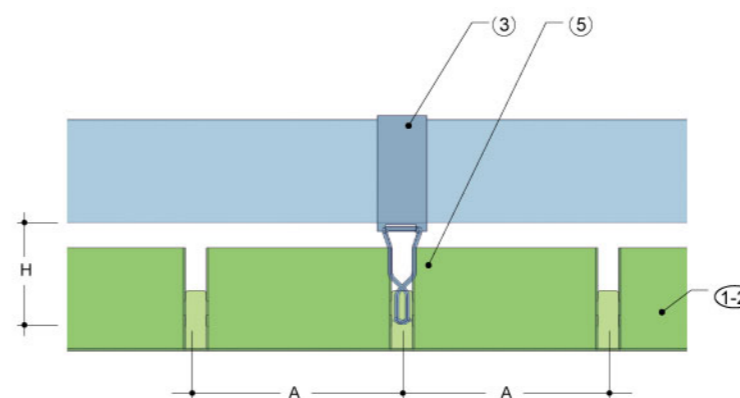
图2: 格栅系列金属吊顶剖面
