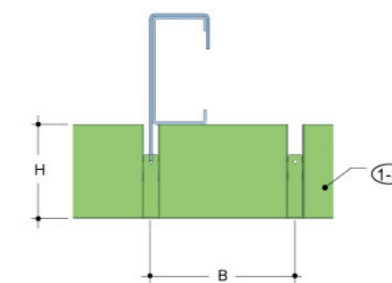
图3: 格栅系列金属吊顶剖面
