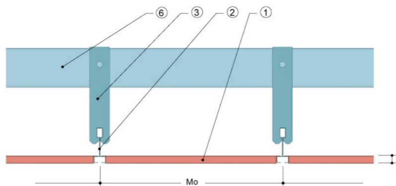
图2: 明架矩形板系列金属吊顶剖面
