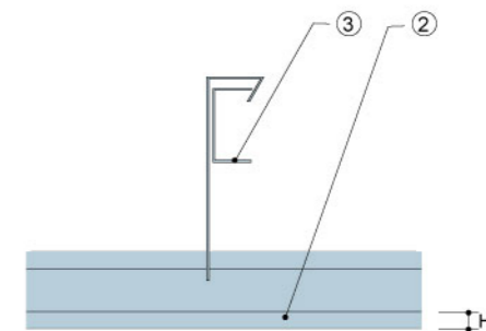
图3: 明架矩形板系列金属吊顶剖面
