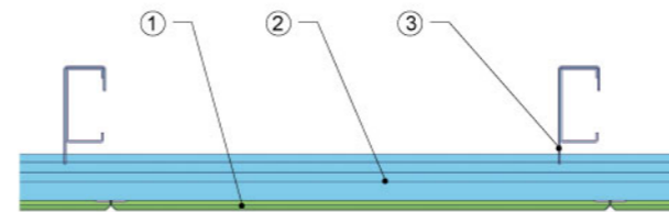
图2: 暗架矩形系列金属吊顶剖面
