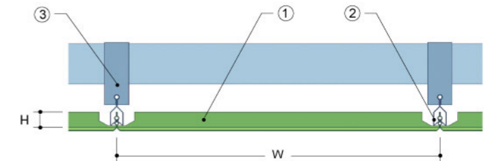
图3: 暗架矩形系列金属吊顶剖面
