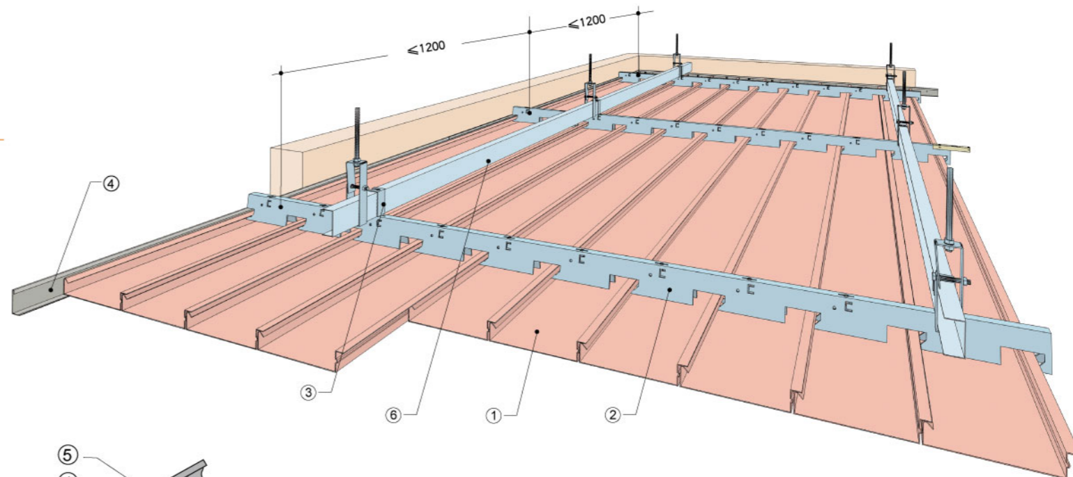
图1: F297H30条型金属吊顶典型的安装尺寸示意图
