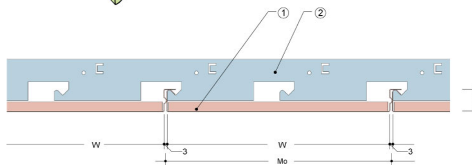
图2: F297H30条型金属吊顶剖面
