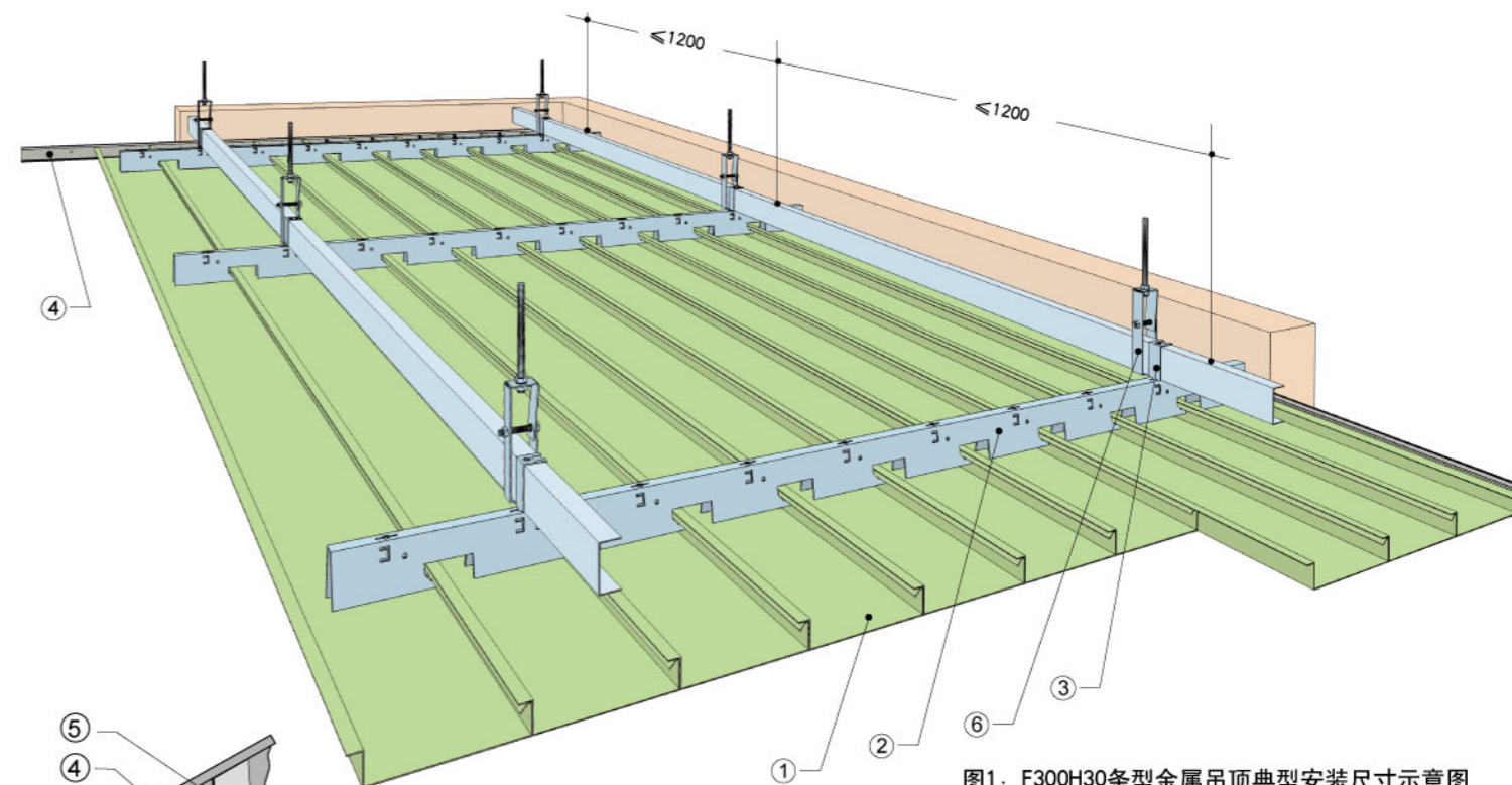
图1: F300H30条型金属吊顶典型安装尺寸示意图
