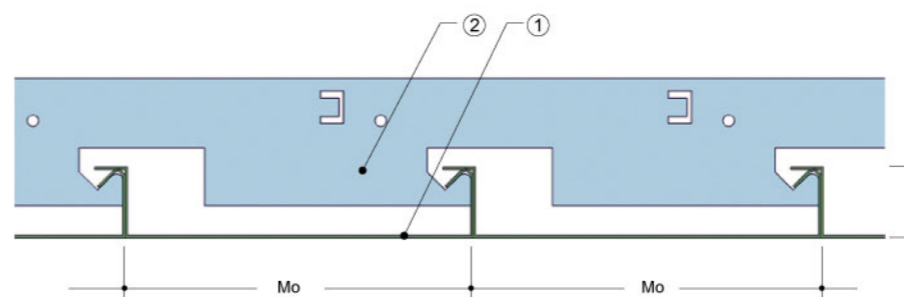
图2: F300H30条型金属吊顶剖面
