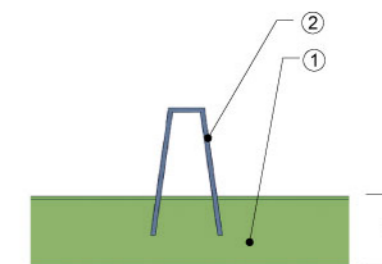
图3: F300H30L条型金属吊顶剖面
