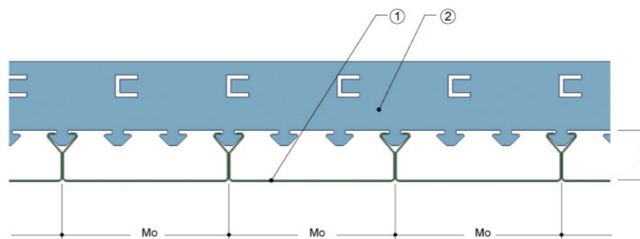
图2: HKF系列条型金属吊顶剖面
