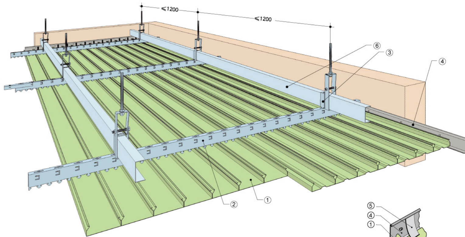
图1: HKF系列条型金属吊顶典型的安装尺寸示意图
