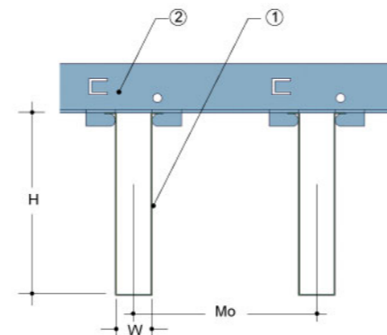
图2: U系列挂片金属吊顶剖面
