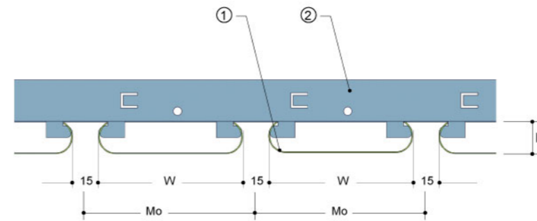
图2: P系列弧型金属吊顶剖面
