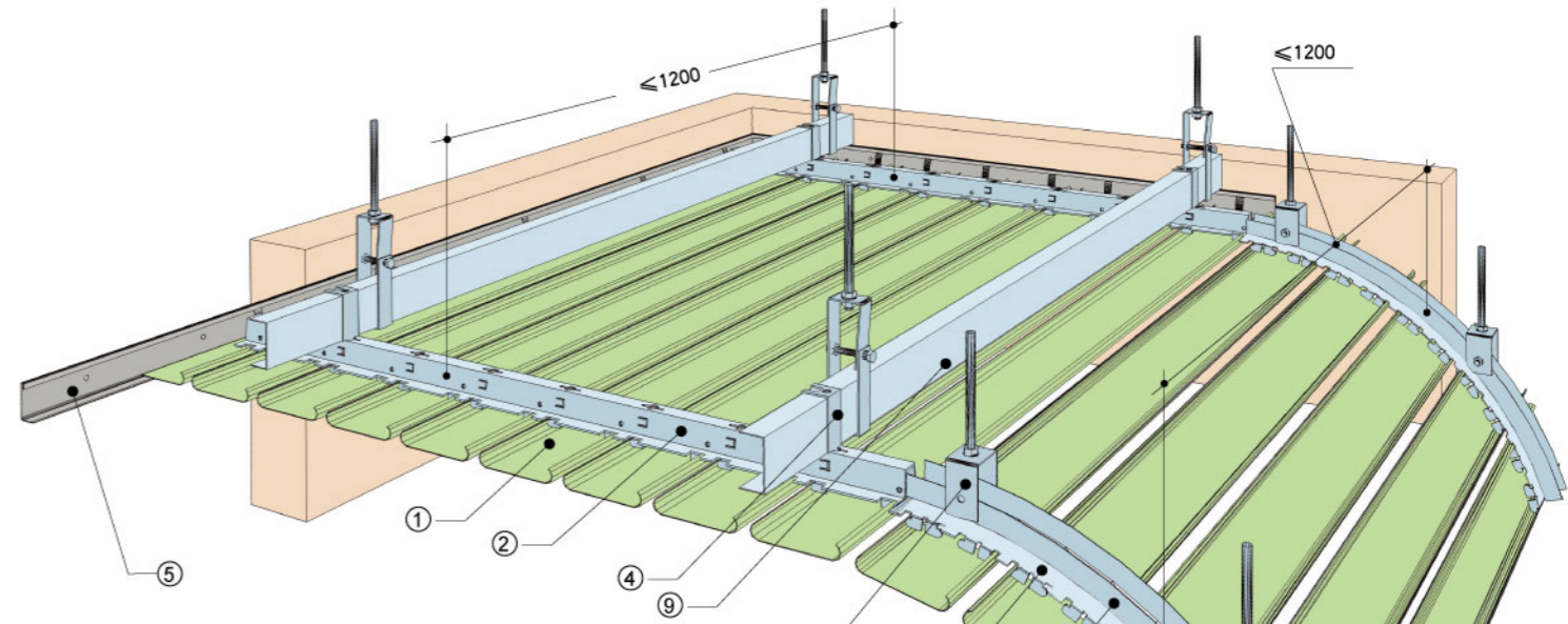
图1: P系列条型金属吊顶典型的安装尺寸示意图
