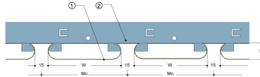
图2: P系列条型金属吊顶剖面
