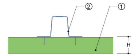
图3: P系列条型金属吊顶剖面
